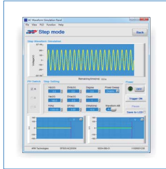
Step mode界面
